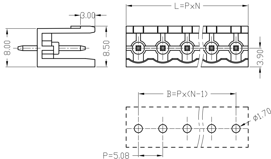
PCB孔位尺寸
